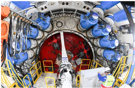
▲ 中铁十四局技术人员在甬舟铁路金塘海底隧道“甬舟号”盾构机内作业。 新华社记者 黄宗治 摄
