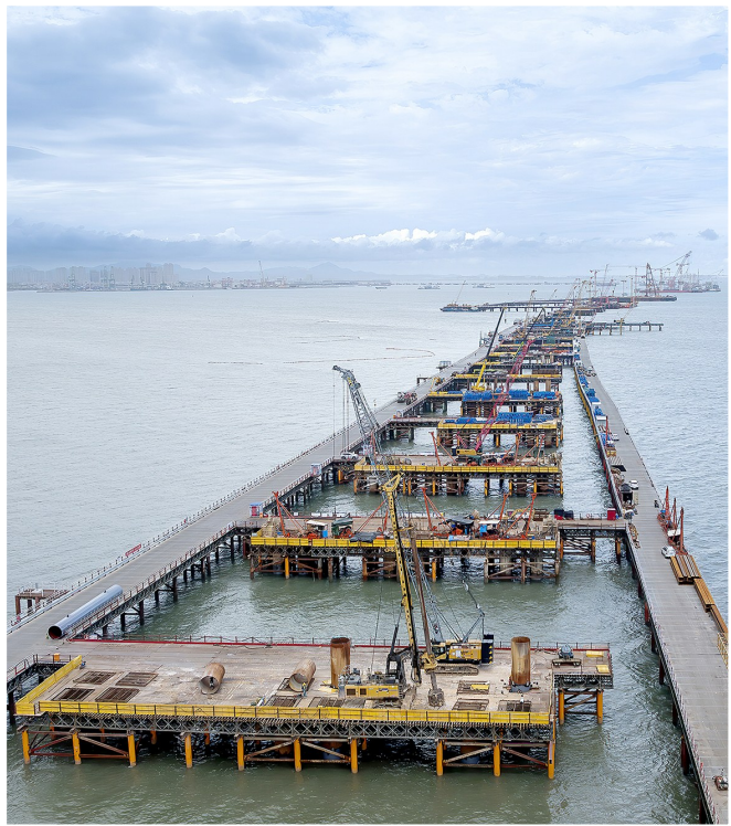
↑ 厦金大桥（厦门段）海上桥梁大规模装配化施工现场（无人机照片，6月13日摄）。
