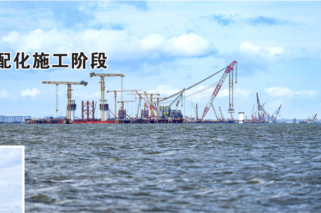
↑ 厦金大桥（厦门段）海上桥梁大规模装配化施工现场（6月13日摄）。
