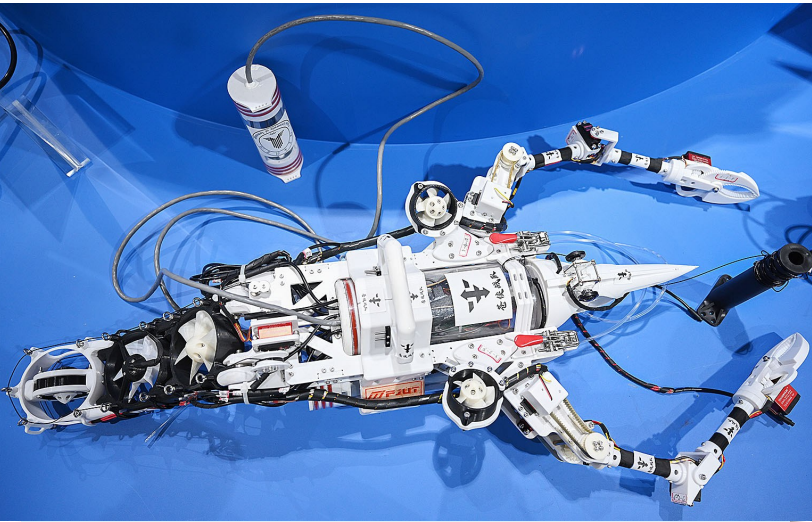
这是11月15日在2024第二届中国海洋装备博览会上拍摄的福建理工大学研发的仿生波士顿大龙虾民用潜航机器人,设备能自动化水下维修检查,有助于潜水探索、水质监测、养殖管理等。11月15日,2024世界航海装备大会在福建福州开幕。 新华社记者 周义 摄
